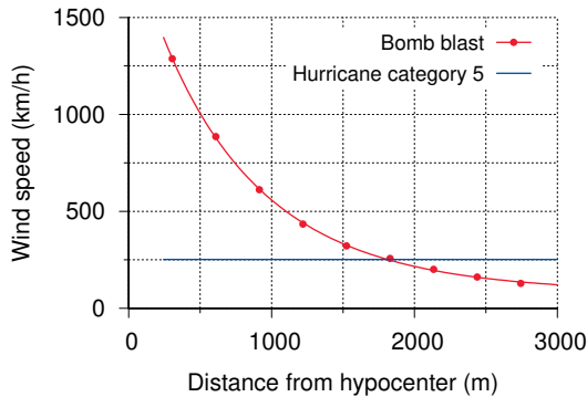
Abbildung 13.2 Windgeschwindigkeit der Druckwelle einer “nominalen” Atombombe. Datenpunkte aus Tabelle 5.45 in [48]. Die Windgeschwindigkeit eines Hurrikans der Kategorie 5 ist zum Vergleich gezeigt.
