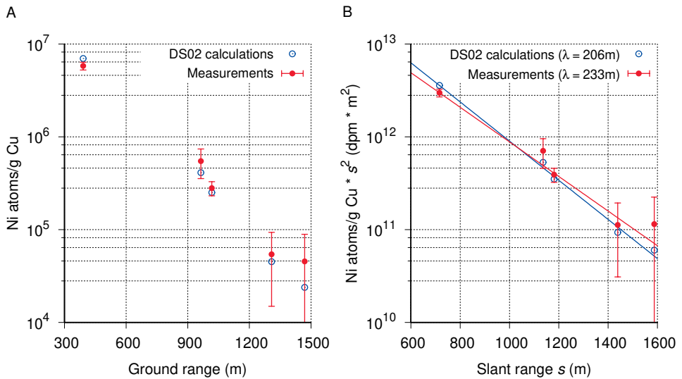
Abbildung 6.8 Messungen der schnellen Neutronenfluenz in Hiroshima durch ^{63}\text{Ni} induziert in metallischen Kupferproben. A: Replot von Abbildung 2 von Seite 677 im DS02 Bericht [85]. B: Analyse der Daten in A nach Gleichung 2.10. Die \lambda -Werte werden aus den Steigungen der angepassten Linien ermittelt. Die Schrägdistanzen wurden aus den Bodenentfernungen nach Gleichung 6.2 berechnet, unter Verwendung einer Detonationshöhe von 600 m.
