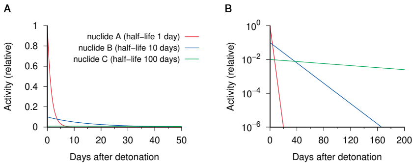
Abbildung 2.2 Zeitlicher Verlauf der Aktivität für drei hypothetische Nuklide mit unterschiedlichen Halbwertszeiten. Zum Zeitpunkt Null sind die Mengen der Nuklide A-C identisch, aber die Aktivität ist für das Nuklid A, das die kürzeste Halbwertszeit hat, am höchsten. Nach drei Wochen ist A jedoch praktisch verschwunden, und nach 200 Tagen ist nur noch das Nuklid C in nennenswerten Mengen vorhanden. Die Tafeln A und B stellen die gleichen hypothetischen Zerfälle dar, aber das semilogarithmische Format in B zeigt Aktivitäten mit sehr unterschiedlicher Größenordnung besser an.
