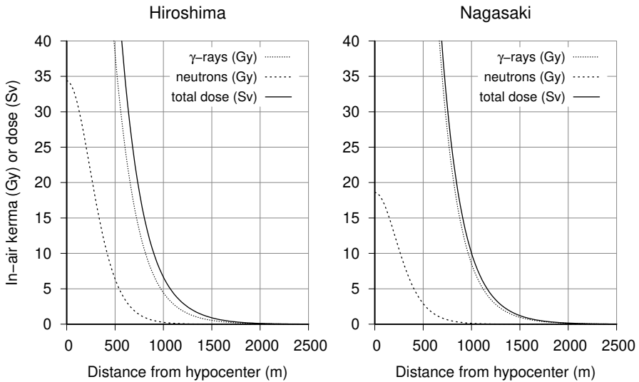
Abbildung 8.1 Geschätzte Strahlungsdosen in Hiroshima und Nagasaki, als Funktion der Entfernung vom Hypozentrum. Die Werte für das Kerma im Freien (“in-air kerma”) für \gamma -Strahlen und Neutronen wurden aus Cullings u. a. [29] entnommen. Um die Gesamtdosis zu berechnen, wurde die dosisabhängige relative biologische Effektivität der Neutronen nach Sasaki u. a. [46] geschätzt (siehe Text für weitere Details).
