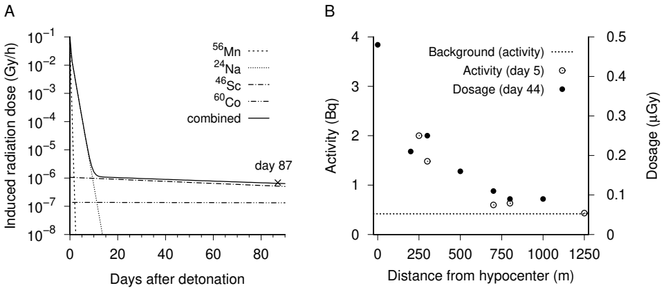
Abbildung 4.1 Schätzungen und Messungen der induzierten Radioaktivität in Hiroshima. A: Induzierte Radioaktivität im Hypozentrum als Funktion der Zeit, extrapoliert von einem einzigen gemessenen Datenpunkt (Tag 87) nach Okajima u. a. [28]. Die durchgezogene Linie ist die Summe aller individuellen Isotopenaktivitäten. Siehe Text für weitere Erklärungen. B: Zwei Datenreihen, die von Takeshita [75] gezeigt werden. Die Maße nach 5 Tage sind in Bq angegeben, während die am Tag 44 in \mu\text{Gy} angegeben sind.
