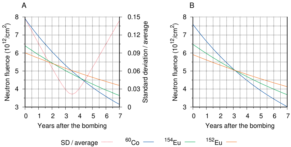
Abbildung 6.7 Abschätzung des Datums der Neutronenaktivierung durch Vergleich der Fluenzen für verschiedene Isotope. A: Geschätzte Neutronenfluenz von ^{60}\text{Co} , ^{152}\text{Eu} , und ^{154}\text{Eu} . Die Schätzungen der drei Isotope weichen zum Zeitpunkt des Bombenangriffs voneinander ab, aber sie ähneln sich, wenn man sie auf 3,5 Jahre später projiziert; dies ist also der wahrscheinlichste Zeitpunkt der Neutroneneinwirkung. B: Neuberechnung der Fluenzschätzungen aufgrund von Aktivitäten, die ebenfalls in [90] angegeben sind. Siehe Text für weitere Details.
