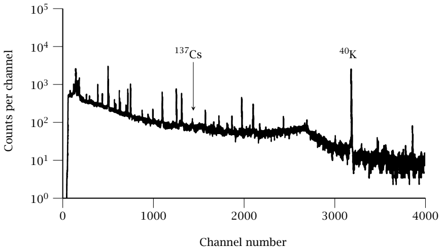
Abbildung 3.3 \gamma -Strahlungs-Spektrum, gemessen von Shizuma u. a. [59] an einer der Proben, die am 9. August 1945 von Yoshio Nishina gesammelt wurden. Der ^{137}\text{Cs} Peak ist auf Fallout zurückzuführen, während der ^{40}\text{K} Peak Teil des natürlichen Hintergrundes ist.
