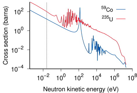
Abbildung 2.3 Neutroneinfangsquerschnitte von ^{59}\text{Co} und ^{235}\text{U} , in Abhängigkeit von der kinetischen Energie der Neutronen. Der Querschnitt hat die Dimension einer Fläche, misst aber eigentlich die Wahrscheinlichkeit des Einfangens. Die schwarz gepunktete Linie gibt die typische Energie eines thermischen Neutrons an (0.025 eV). Die Daten stammen aus [42].
