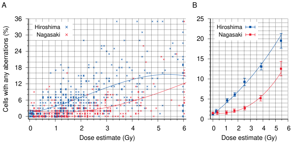
Abbildung 11.3 Chromosomenaberrationen in peripheren Blutlymphozyten, die bei Überlebenden der Atombombe beobachtet wurden. A: Zellen mit Aberrationen, beobachtet bei einzelnen Überlebenden aus Hiroshima und Nagasaki, aufgetragen gegen T65D Strahlungsdosis-Schätzungen [215]. Trendlinien sind Polynome dritter Ordnung; beide haben R^2 -Werte nahe 0,34. B: Dieselben Daten wie in A, nach der Verarbeitung in RERFs Schlichterei Statistikabteilung (Reproduktion von Abbildung 3 in Otake [215]). Der Autor bezeichnet seine Fehlerbalken als “95% Konfidenzintervalle”.
