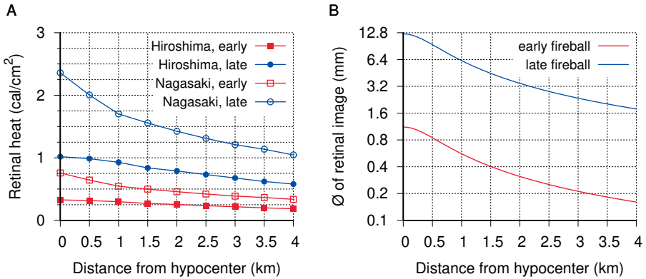
Abbildung 10.4 Thermische Energiedichte (A) und Durchmesser (B) der Netzhautbilder der Atombomben von Hiroshima und Nagasaki. Die Markierungen ‘early’ und ‘late’ in A beziehen sich auf das Stadium des Feuerballs. Siehe Text für weitere Details.
