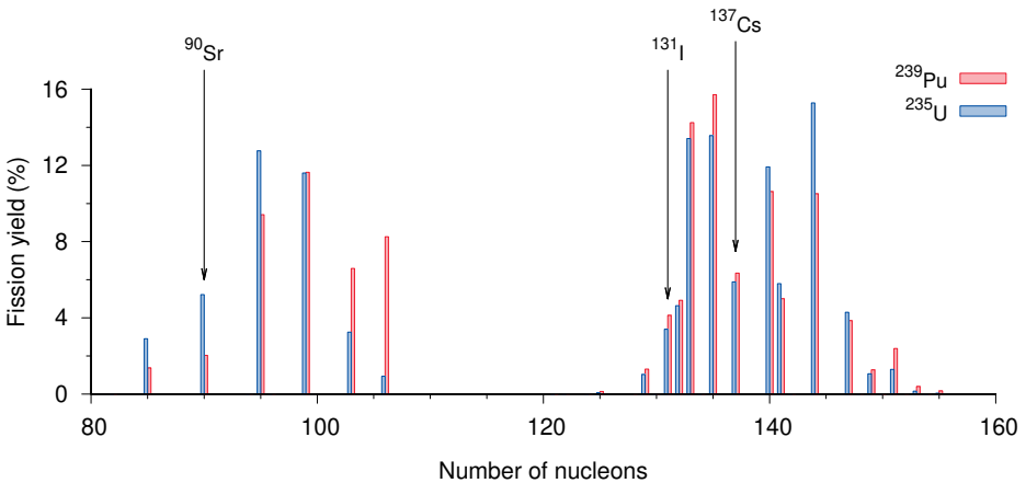
Abbildung 2.4 Spaltprodukte von ^{239}\text{Pu} und ^{235}\text{U} unter der Einwirkung von schnellen Neutronen. Nuklide mit der gleichen Anzahl von Nucleonen wurden in dieser Grafik zusammengefasst, aber die drei hervorgehobenen Nuklide sind jeweils die einzigen mit der betreffenden Nucleonenzahl. ^{90}\text{Sr} ähnelt chemisch dem Kalzium und sammelt sich im Knochen an, während ^{131}\text{I} sich in der Schilddrüse ansammelt. ^{137}\text{Cs} ähnelt dem Kalium und kann sich diffus in allen Geweben anreichern. Außerdem wird es auch häufig als Marker für nuklearen Fallout in der Umwelt verwendet. Daten aus [44].
