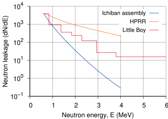
Abbildung 6.2 Neutronen-Quellspektrum der Hiroshima-Bombe nach Loewe und Mendelsohn [84]. Die beiden anderen gezeigten Spektren stellen plausible Grenzfälle für das Bombenspektrum dar; alle drei wurden willkürlich bei einer Neutronenenergie von 0.6 MeV auf den gleichen Wert normiert. Im T65D-Dosimetrie-Schema wurde angenommen, dass das Spektrum der Hiroshima-Bombe (“Little Boy”) dem des “Health Physics Research Reactor” (HPRR) ähnelt; das hier gezeigte “Little Boy”-Spektrum wurde von Loewe und Mendelsohn vorgeschlagen.
