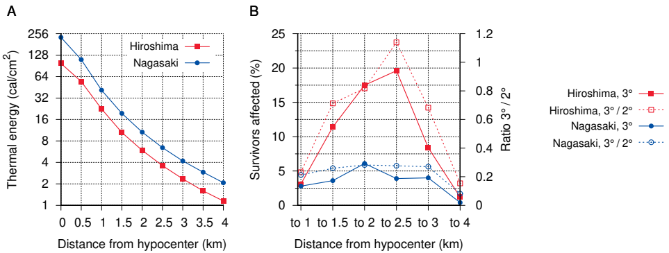
Abbildung 9.1 Strahlungshitze und Verbrennungen bei unterschiedlichen Entfernungen von den Hypozentren in Hiroshima und Nagasaki. A: Strahlungswärme (Kalorien pro \text{cm}^2 ) vs. Entfernung vom Hypozentrum. Daten aus Ishikawa u. a. [8]. B: Inzidenz von Verbrennungen dritten Grades bei Opfern, die 20 Tage nach den Bombenangriffen noch am Leben waren, nach Entfernung vom Hypozentrum, und Verhältnis der Inzidenz von Verbrennungen dritten Grades zu denen zweiten Grades. Patienten mit Verbrennungen sowohl zweiten als auch dritten Grades werden nur in der letzteren Kategorie gezählt. Daten aus [32, Tabellen 9H und 9N].
