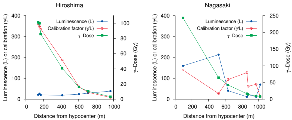
Abbildung 5.4 Proben-Thermolumineszenz, Kalibrierungsfaktoren und \gamma -Dosen vs. Entfernung von den Hypozentren in Hiroshima und Nagasaki. Alle Daten sind aus Tabelle 2 im Hashizume u. a. [78]. In der Studie sind keine Einheiten für die Lumineszenzmesswerte und Kalibrierungsfaktoren angegeben; die \gamma -Dosen sind im Original in rad angegeben, wurden hier aber in Gy umgerechnet.
