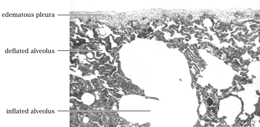
Abbildung 10.6 Lungenemphysem (übermäßige Inflation) und Atelektase (übermäßige Deflation) bei einem frühen Todesfall aus Hiroshima. Fotografie aus Liebow u. a. [41], Beschriftungen von mir.
