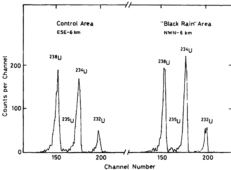
Abbildung 3.2 \alpha -Strahlungs-Spektren von Uran, das aus Bodenproben mithilfe von 0.1 N Salpetersäure extrahiert wurde (entnommen aus Takada u. a. [55]). Die \alpha -Teilchen, die von den verschiedenen Uranisotopen emittiert werden, unterscheiden sich durch ihre charakteristischen Energien, die "Kanälen" entlang der x -Achse entsprechen; die Häufigkeit jedes Isotops wird durch die Fläche unter seinem Peak dargestellt (und nicht durch die dessen Höhe). Siehe Text für weitere Details.
