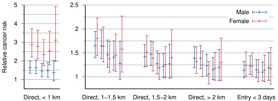
Abbildung 12.7 Krebsrisiko bei Personen, die direkt dem Bombenangriff in Hiroshima ausgesetzt waren und bei früh in die Stadt Gekommenen. Daten aus Tabelle 5 in Matsuura u. a. [258]. Direkt exponierte Subjekte werden nach der Entfernung vom Hypozentrum gruppiert; eine fünfte Gruppe umfasst diejenigen, die zwischen dem 6. und 8. August in die Nähe des Hypozentrums (<2 km) kamen. In jeder Gruppe repräsentieren die fünf Werte (mit 95% Konfidenzintervallen) die Sterberaten für die Beobachtungszeiträume ab dem 1. Januar 1968, 1971, 1974, 1977 und 1980. Ein Risiko von 1,0 wurde denen zugeschrieben, die nach > 3 Tagen in die Stadt kamen.
