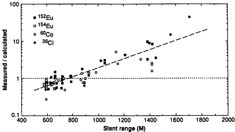
Abbildung 6.4 Verhältnis von gemessener zu berechneter Neutronenaktivierung als Funktion der Entfernung vom Epizentrum (“Slant range”). Darstellung aus Abbildung 1 in Straume u. a. [94]. Die Berechnung der erwarteten Neutronenaktivierung wurde von diesen Autoren nach dem damals aktuellen DS86-Dosimetrieschema durchgeführt. Die Autoren nahmen ihre Datenpunkte aus insgesamt zehn verschiedenen Studien, die wie angegeben verschiedene Isotope verwendeten.
