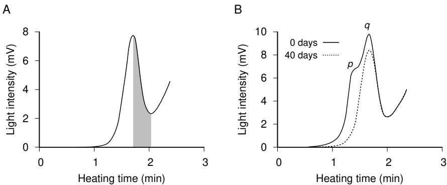
Abbildung 5.1 Thermolumineszenz-Kurven von Ziegel- oder Kachelproben, gezeichnet nach Abbildungen 6 (A) und 10 (B) in Hashizume u. a. [78]. Die Proben wurden innerhalb von 3 min von Umgebungstemperatur auf 300°C erhitzt. A: Beschrieben als “eine typische Thermolumineszenz-Glühkurve”, die “von einer Probe erhalten wurde”. Der Teil der Signalkurve, der durch die schattierte Fläche angezeigt wird, wurde zur Bestimmung der absorbierten \gamma -Strahlendosis verwendet. B: Glühkurve einer experimentell bestrahlten Probe, die zwei überlappende Peaks bei ungefähr 1.4 min/140°C ( p ) bzw. 1.8 min/180°C ( q ) zeigt. 40 Tage nach der Bestrahlung ist p verschwunden, während q noch da ist; mit diesem Beleg in der Hand, schätzen Hashizume et al. die Lebensdauer von q auf 670 000 Jahre.
